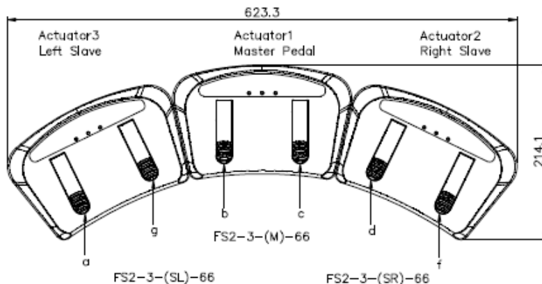
FS2-3-66 Drive3 Actuator
